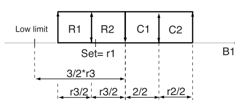
2 resistenze 2 compressori/2 heating elements 2 compr. -Fig. 22/b-
