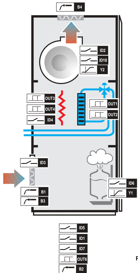
Schema di collegamento / Connection diagram
