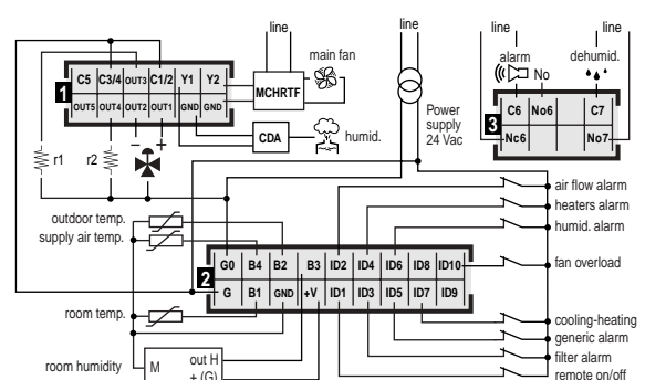
Schema di collegamento / Connection diagram
