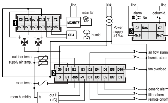
Schema di collegamento / Connection diagram
